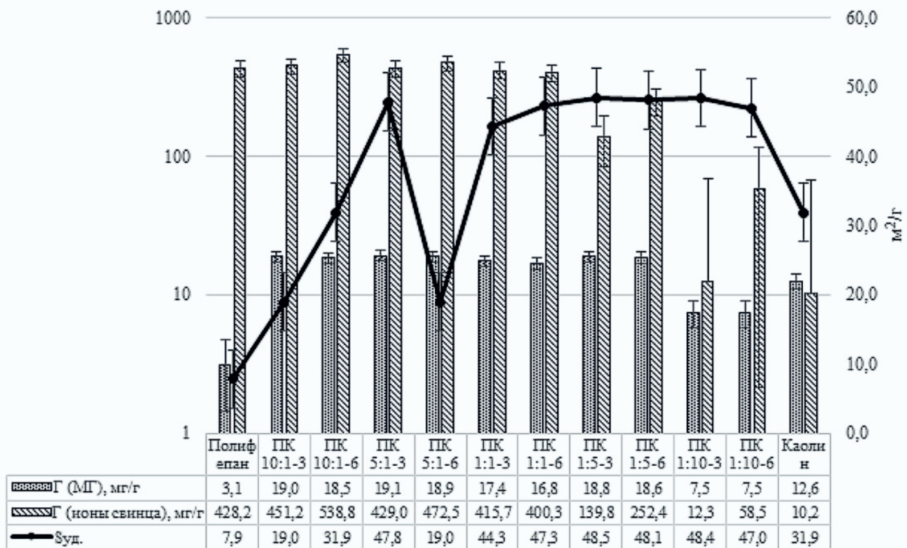
Рисунок 1. Удельная поверхность (м 2 /г) и сорбционная активность (мг/г) каолина, полифосфата и композиционных материалов на их основе по метиленовому голубому и ионам свинца.
